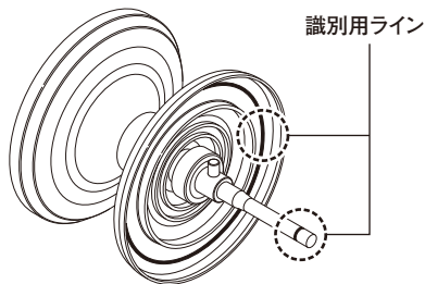
XGモデル スプール組
